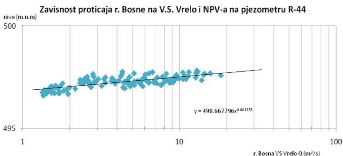
Slika 56. Zavisnost prot. r. Bosne na V.S. Vrelo i NPV-a na pjezometrima P-237, P-220, R-34 i R-44
