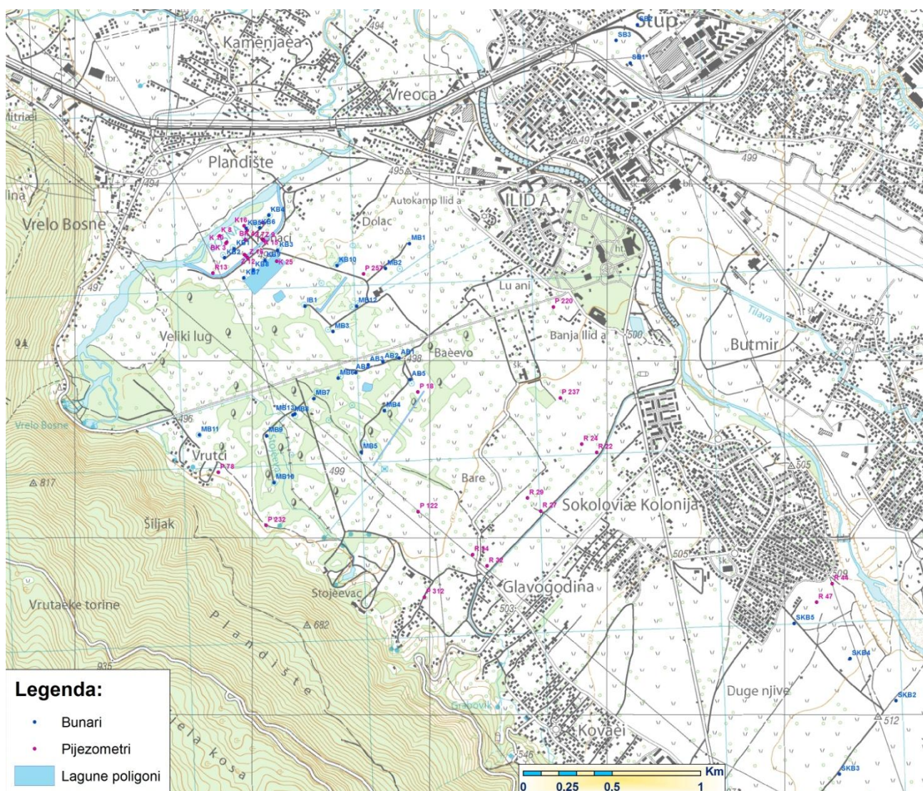
Slika 117. Lokacije objekata u Sarajevskom polju.
