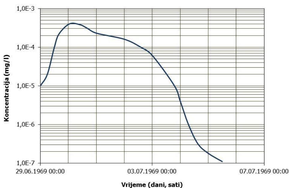
Slika 124. Promjena koncentracije C_{20}H_{10}O_5Na_2 na Vrelu Bosne tokom bojenja izvedenog na ponoru Sitnička lokva
