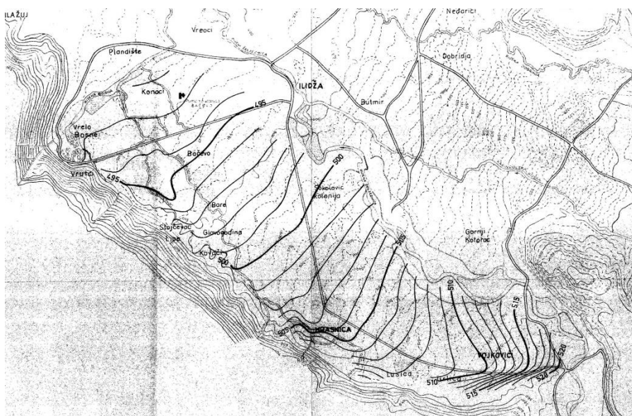
Slika 108. Hidroizohipse minimalnog nivoa podzemne vode u Sarajevskom polju na prostoru Bačovo – Vojkovići za period 1965 – 1969 godine (ZHGF, 1971)
