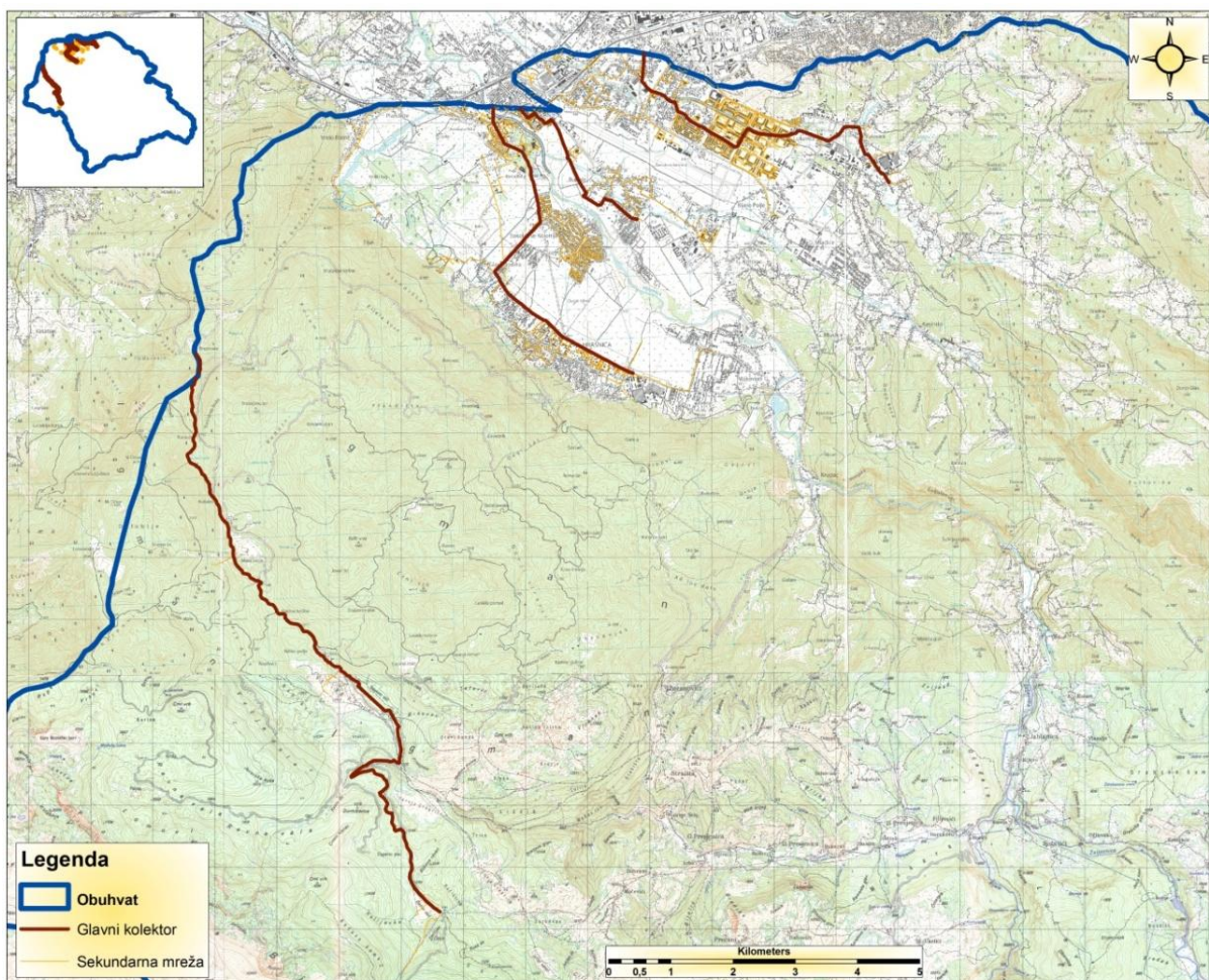
Slika 138 Kolektori i sekundarna mreža
