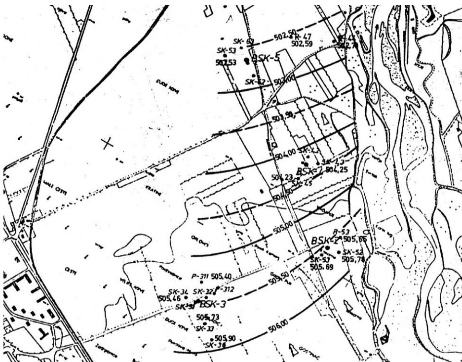
Slika 83. Potencijalne linije na izvišću Sokolović kolonija za dan 06.01.1997. godine, Q_{Z.V.S. ILIDŽA} = 28 \text{ m}^3/\text{s} ,
