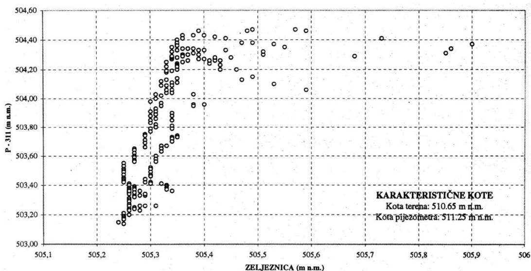
Slika 87. Zavisnost vodostaja na pijezometru P-311 i vodostaja u rijeci Željeznici za period IV/97 – IV/98 (Situacija prije puštanja izvorišta u pogon)
