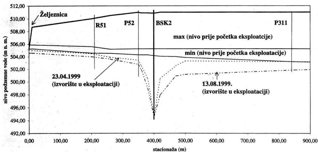
Slika 90. Karakteristični nivoi podzemnih voda na izvorištu Sokolovići
