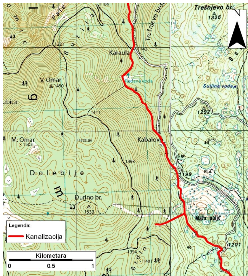
Slika 145. Lokacija Malog polja sa prikazom dijela trase kolektora Šinji do-Hadžići
