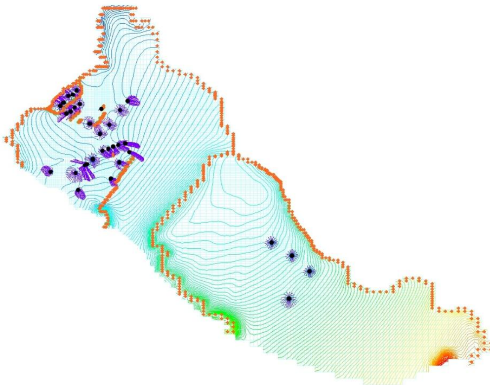
Slika 162. Tečenje 10dana
