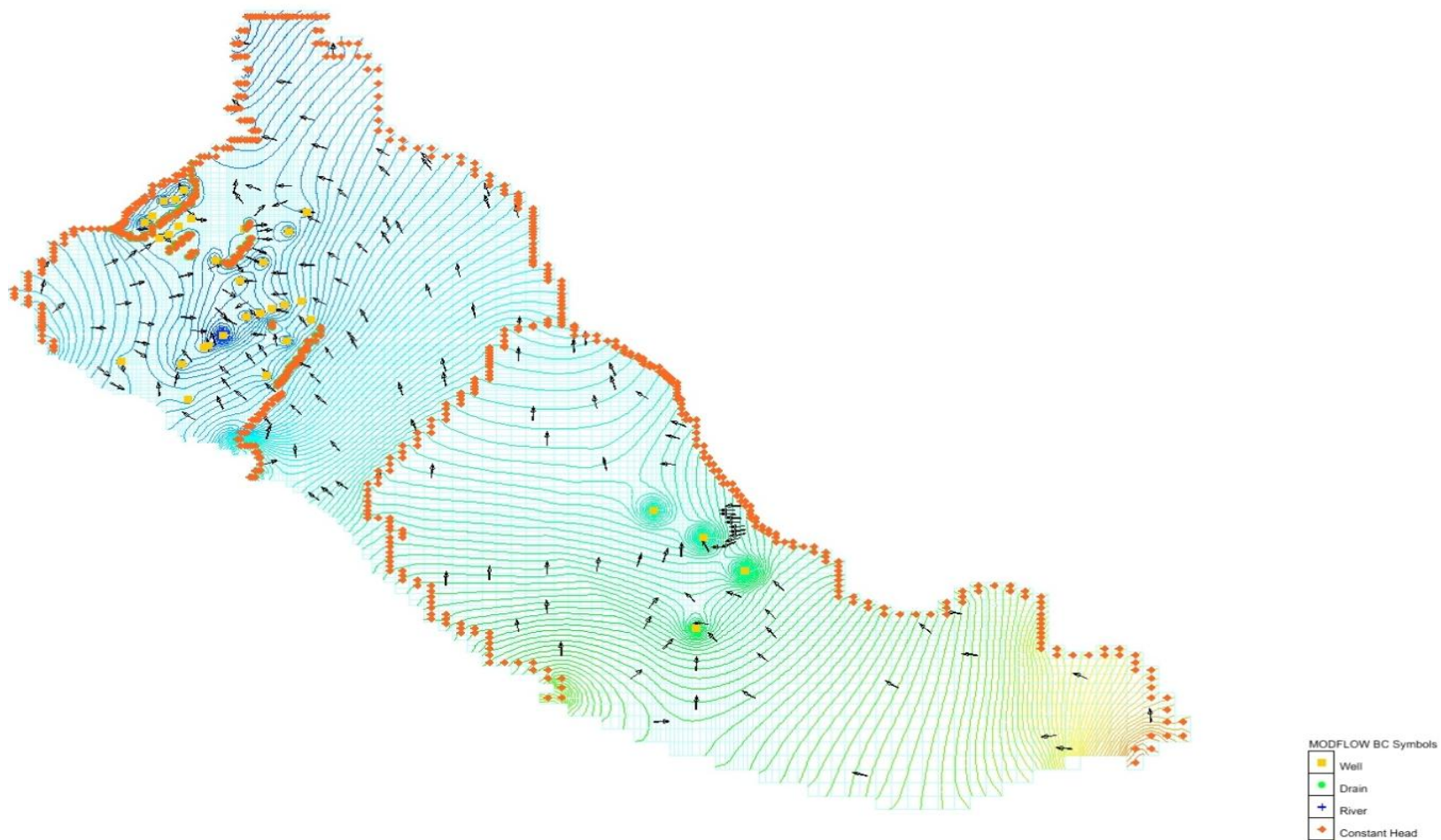
Slika 161. Hidroizohipse-Vektori brzine
