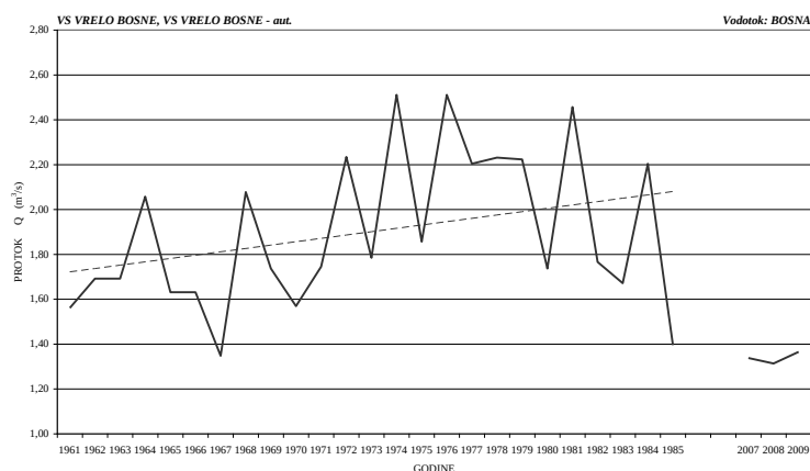
Slika 30. Hidrogram minimalnih godišnjih proticaja
