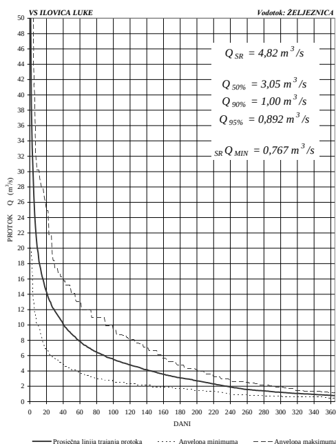
Slika 47. Linija trajanja proticaja r. Željeznice na VS Ilovica Luke sa anvelopama min. i maks. voda
