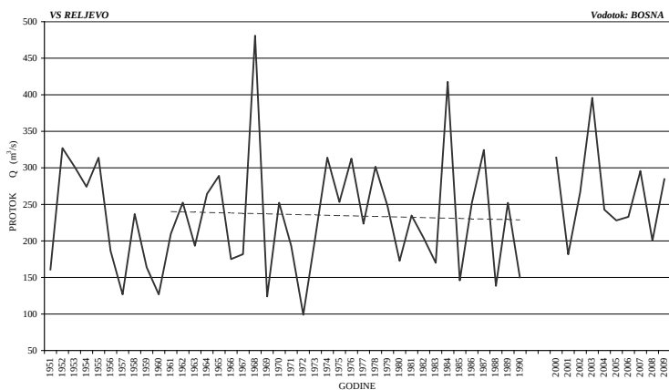
Slika 40. Hidrogram maksimalnih godišnjih proticaja
