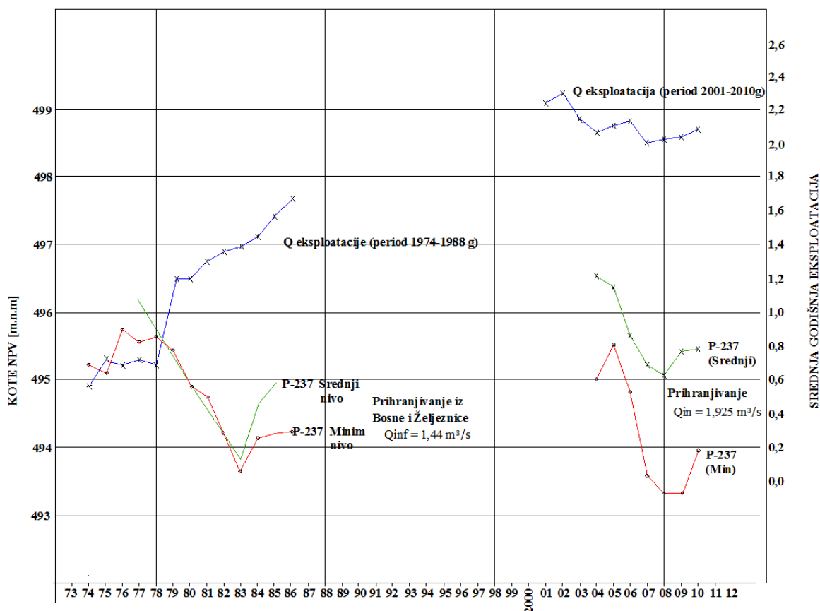
Slika 118. Promjena NPV-a na P-237 u funkciji količine eksploatacije na izvoru u periodu 1974-1986, i u periodu 2004-2010 godina
