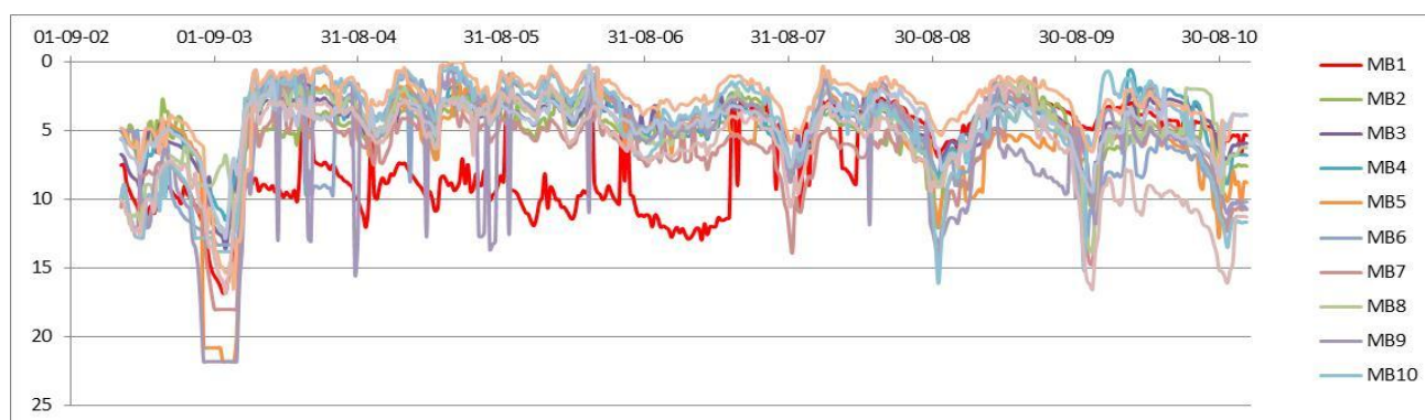
Slika 101. Sniženja nivoa u bunarima MB tokom eksploatacije
