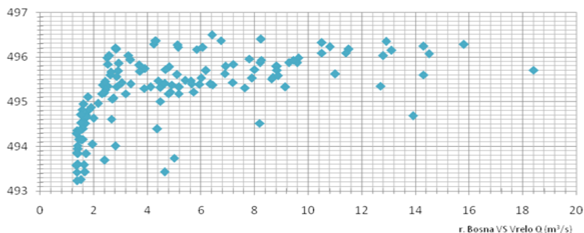
nivo (m.n.m) Zavisnost proticaja r. Bosne na V.S. Vrelo i NPV-a na pjezometru P-237
