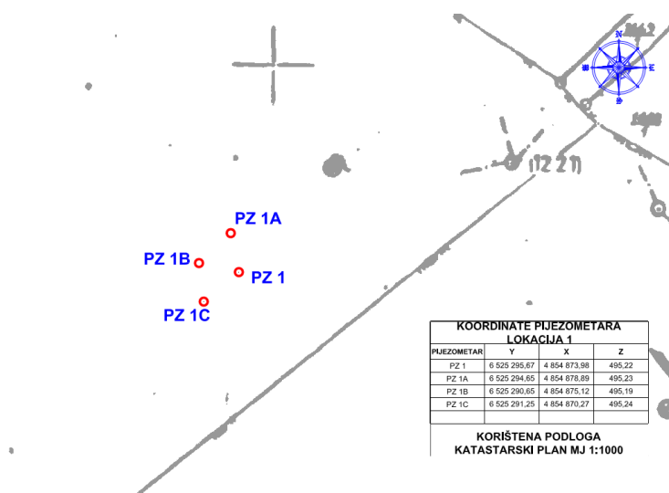
Slika 8. Pozicija pijezometara - Stup
