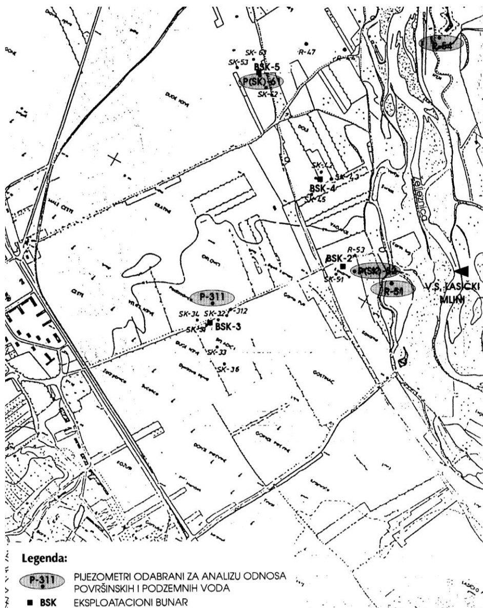
Slika 80. Situacija izvorišta Sokolovići sa pozicijom pijezometara i eksploatacionih bunara za mjerenja infiltracije tokom 1990-tih godina
