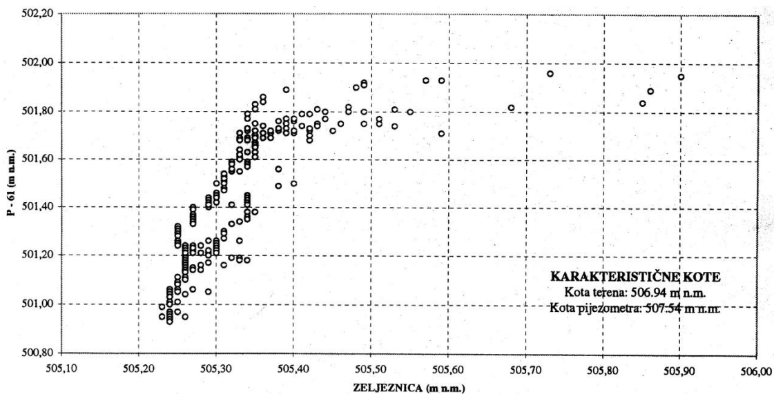
Slika 85. Zavisnost vodostaja na pijezometru P-61 i vodostaja u rijeci Željeznici za period IV/97 – IV/98 (Situacija prije puštanja izvorišta u pogon)
