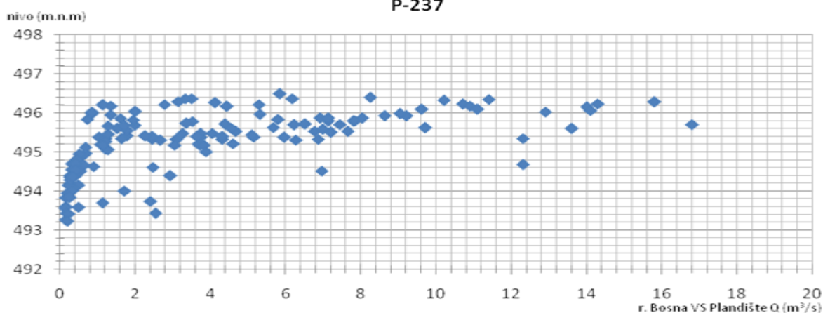
Slika 57. Uspostavljene zavisnosti između proticaja na vodotocima Željeznica v. s. Ilidža te Bosna v.s. Vrelo i Rimski most (Plandište) sa NPV-om na P- 237
