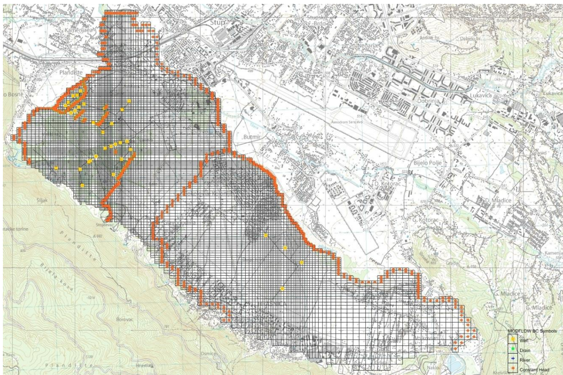
Slika 157. Granični uvjeti
