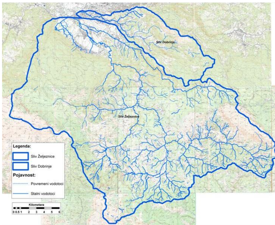
Slika 10. Karta hidrografske mreže na istražnom području izvorišta
