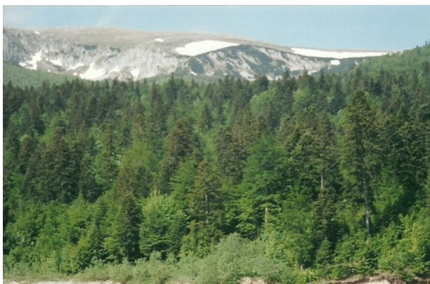
Slika 60. Šumske sastojine u Ravnoj vali, zaostale skupine krivulja na Bjelašnici
