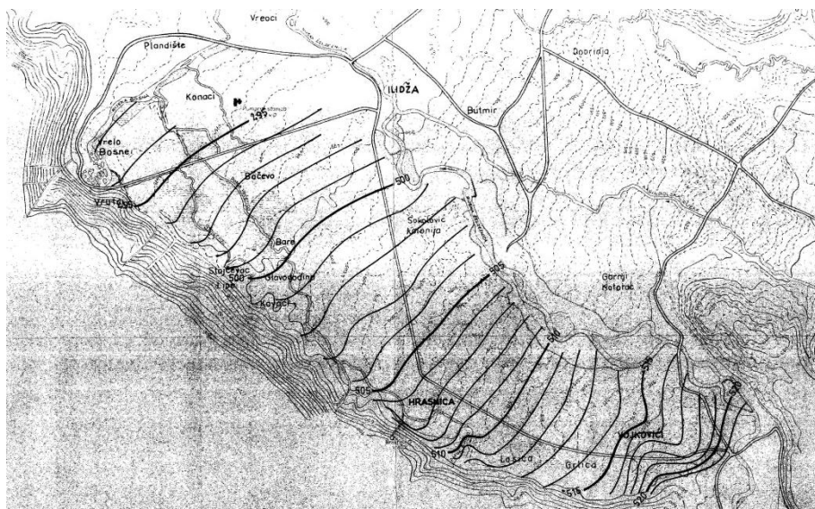
Slika 107. Hidroizohipse maksimalnog nivoa podzemne vode u Sarajevskom polju na prostoru Bačovo – Vojkovići za period 1960 – 1962 godine (ZHGF, 1971)
