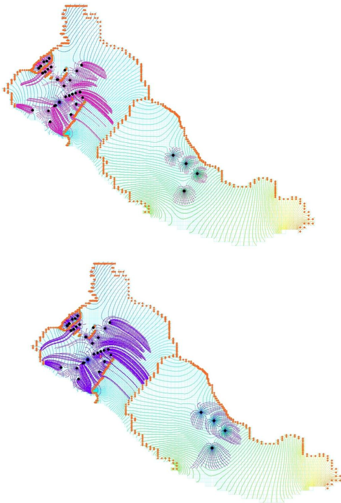
Slika 163. Tečenje 50 dana (gore) i 180 dana (dole)
