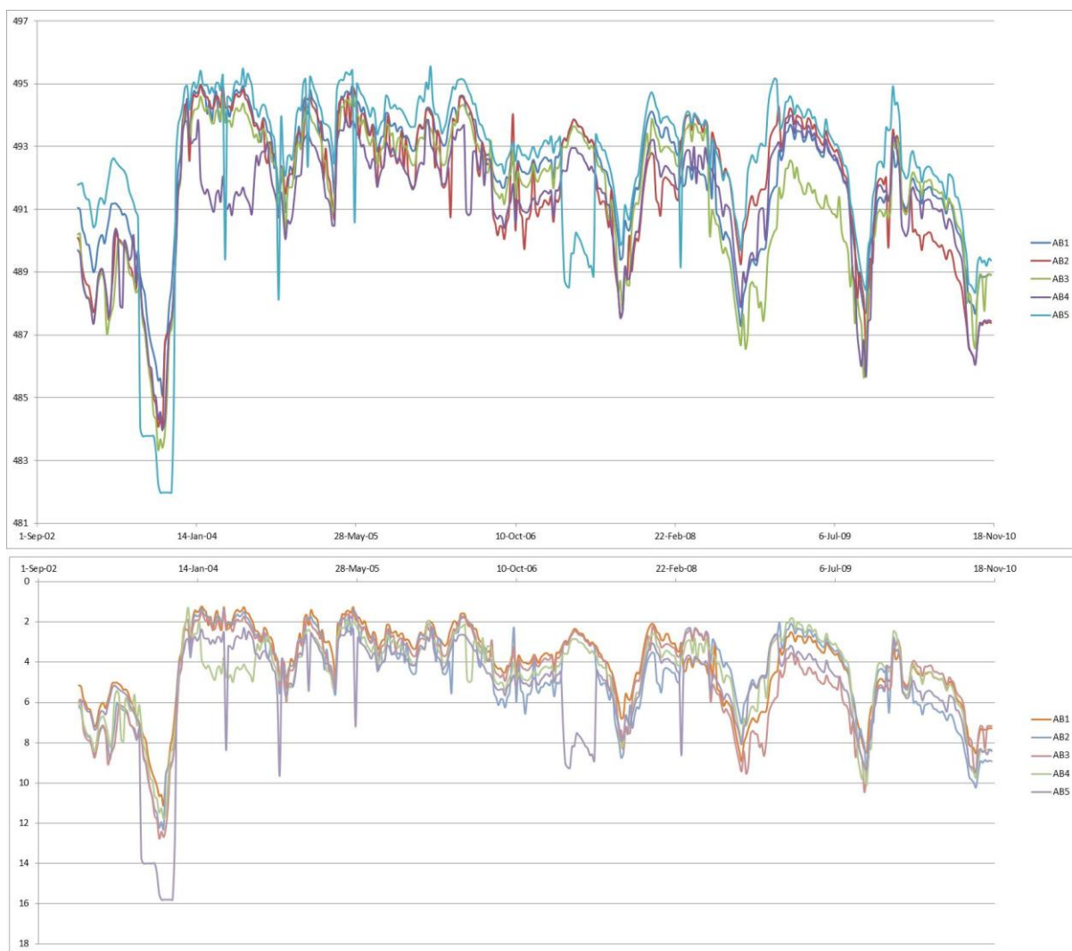
Slika 99. Snižavanja nivoa u bunarima AB tokom eksploatacije
